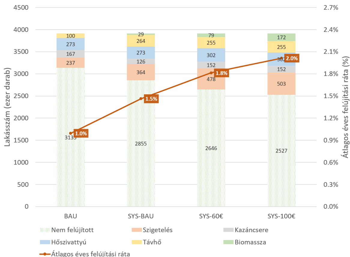
20 ÁBRA: ÉPÜLETFELÚJÍTÁSOK SZÁMA A FELÚJÍTÁS TÍPUSA SZERINT (EZER DARAB) ÉS AZ ÁTLAGOS ÉVES FELÚJÍTÁSI RÁTA VÁLTOZÁSA AZ EGYES FORGATÓKÖNYVEK ESETÉBEN, 2020-2035, (%)
